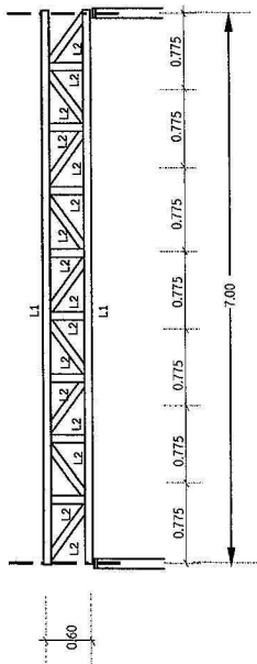
ขยายโครงถัก TRUSS 2 มาตราส่วน 1:150
