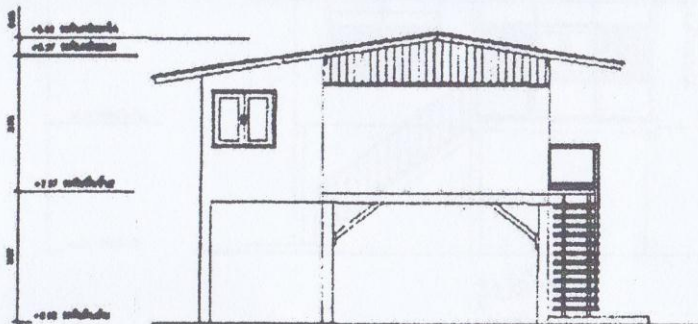
รูปด้าน 1 มาตราส่วน 1:75
