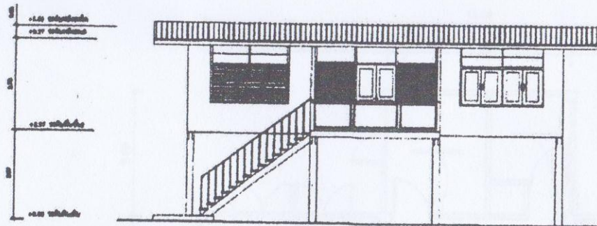
รูปด้าน 3 มาตรฐาน 1:75
