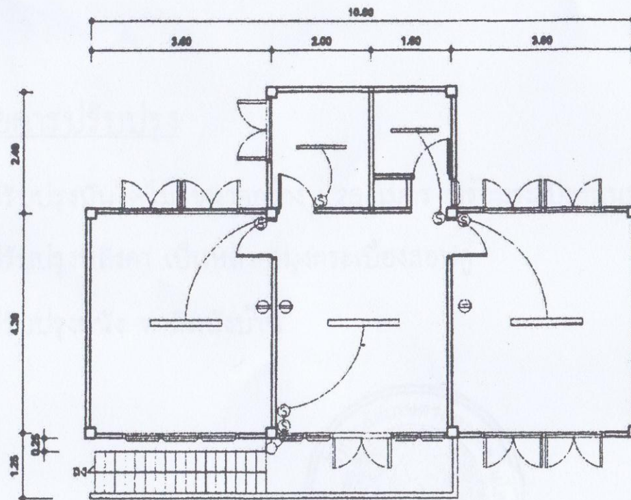
แปลนพื้นและผังไฟฟ้า มาตรฐาน 1:50
