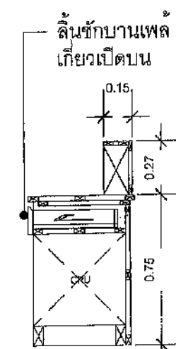
F-03 SECTION 1 : 25
