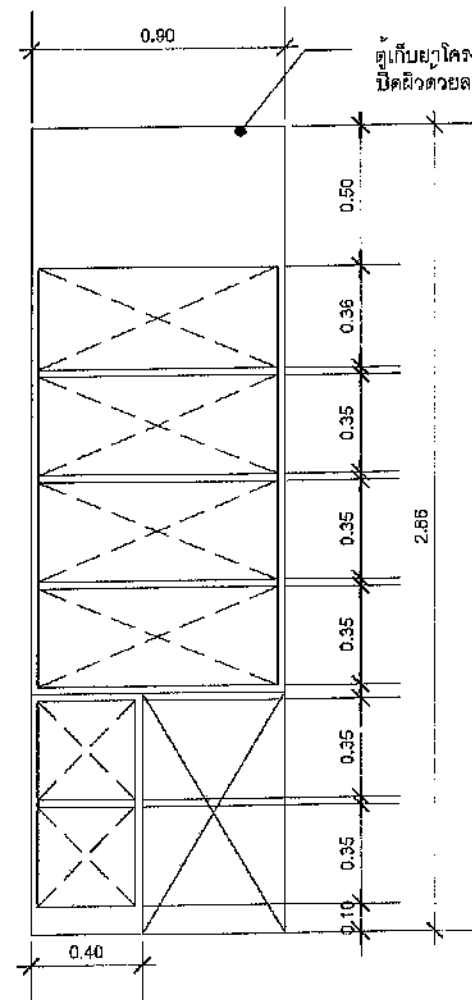
16.3 รูปด้าน 1:25
