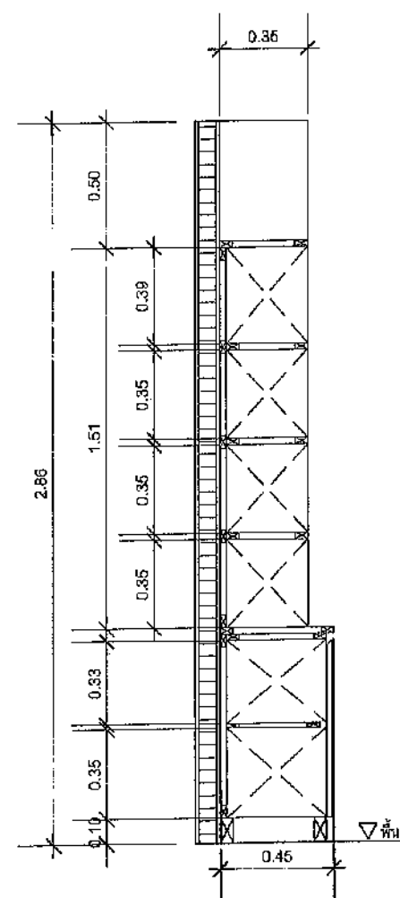
SE20 รูปตัด 1:25
