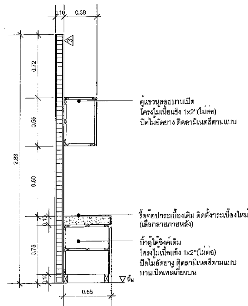
รูปตัด SE11 มาตราส่วน 1:25
