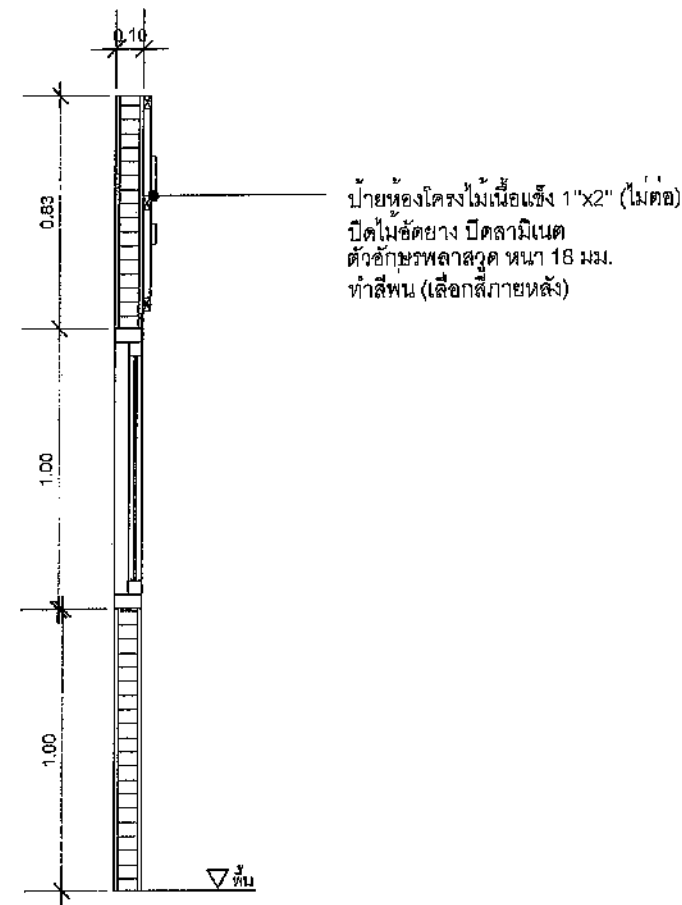
รูปตัด SE9 มาตราส่วน 1:25
