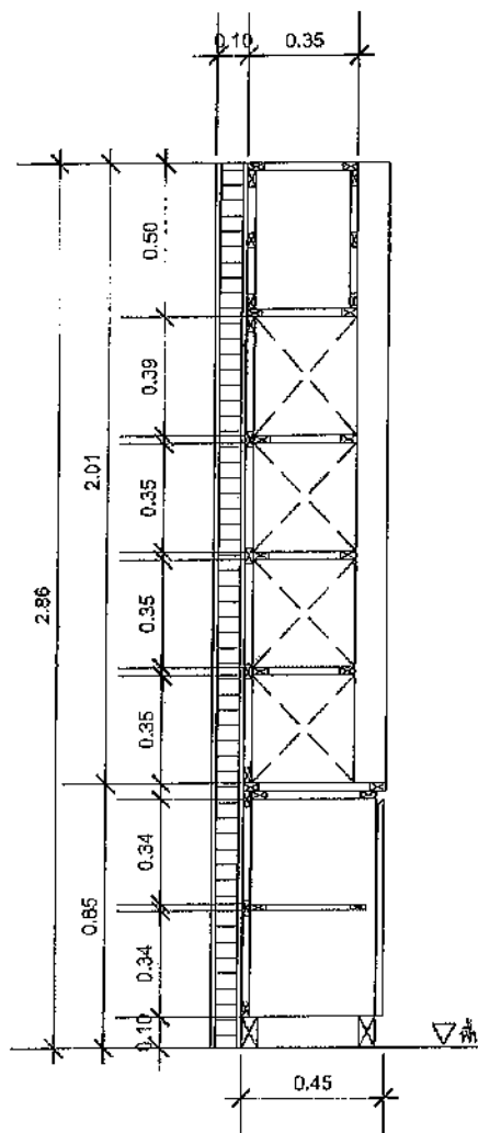
SE18 รูปตัด
