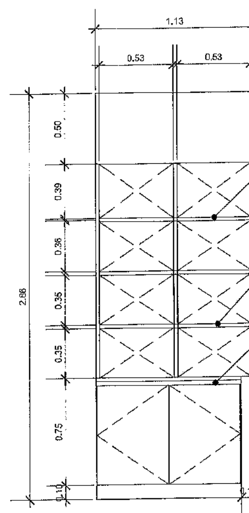
16.1 รูปด้าน 1:25
