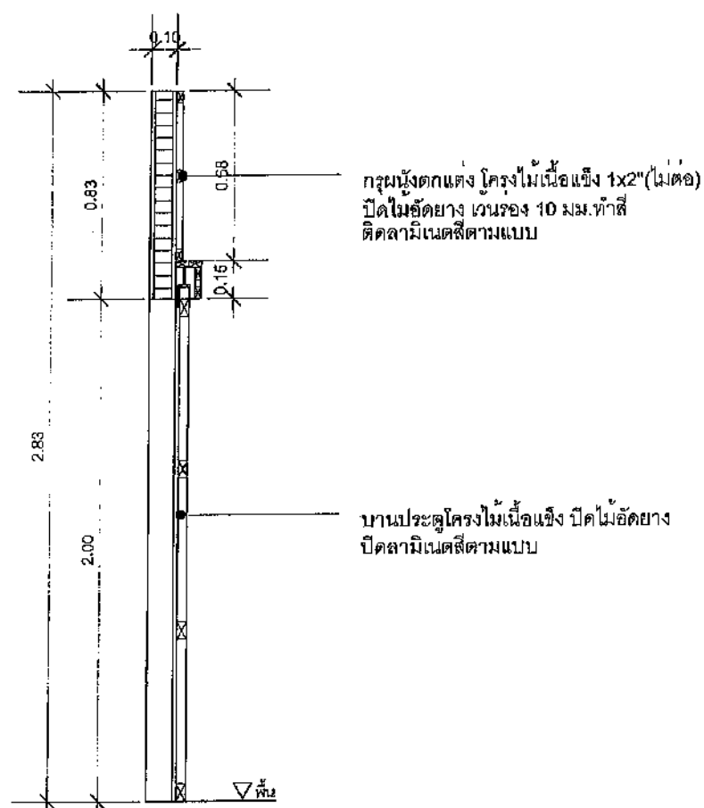
รูปตัด SE8 มาตราส่วน 1:25
