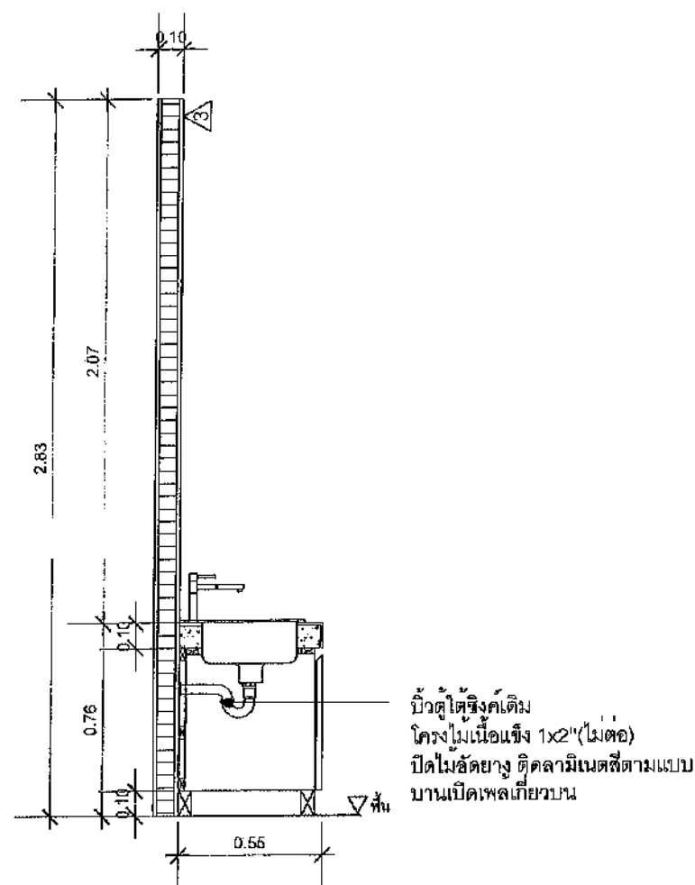
รูปตัด SE10 มาตราส่วน 1:25
