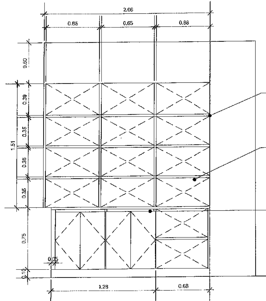
15.2 รูปด้าน
