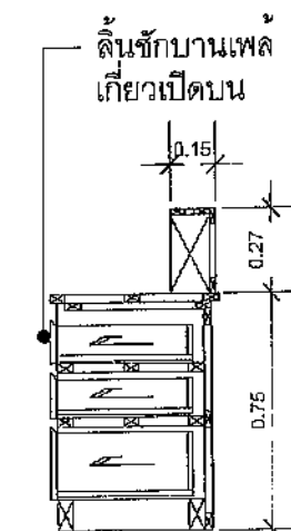
F-04 SECTION 1:25
