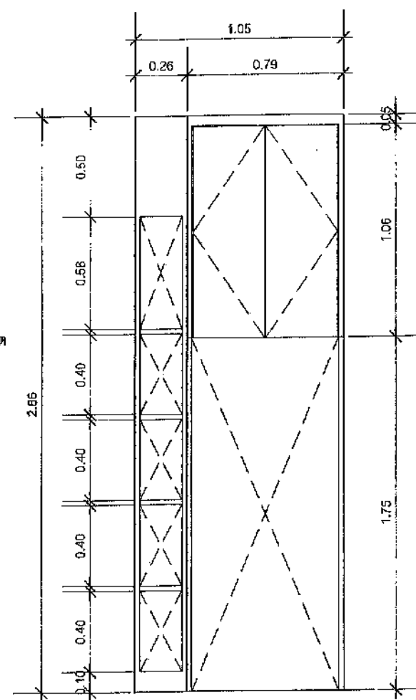
15.3 รูปด้าน 1:25
