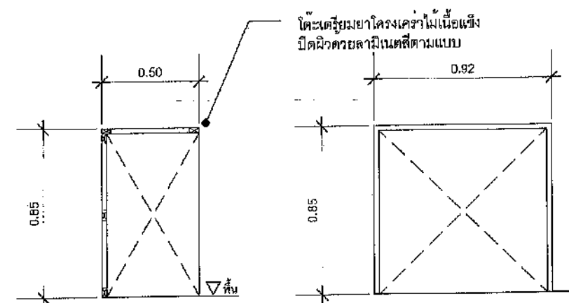
SE23 รูปตัด 1:25
