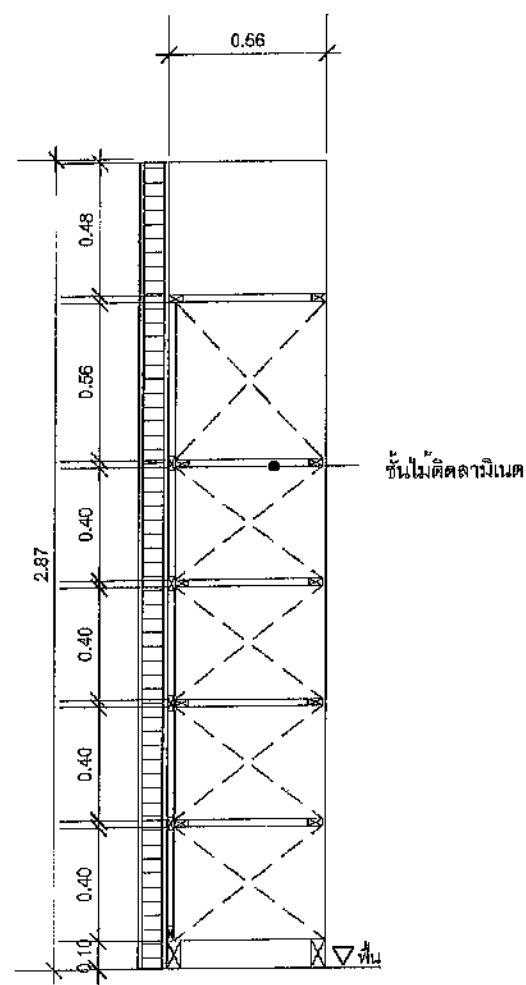
SE19 รูปตัด 1:25
