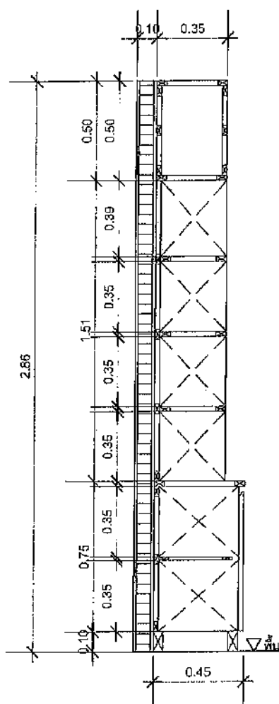
SE17 รูปตัด 1:25
