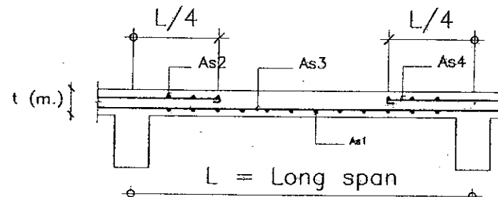
รูปตัดด้านยาว
