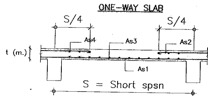
รูปตัดด้านอื่น
