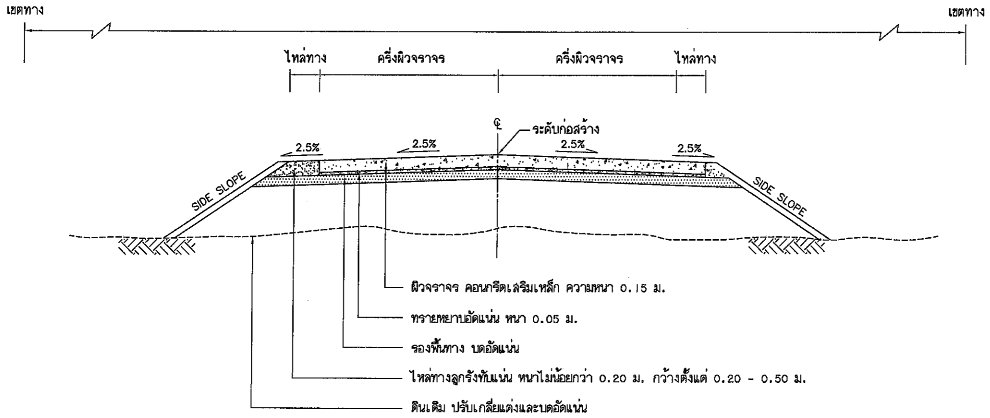
รูปตัดแฉัดของโครงสร้างถนนคอนกรีตเสริมเหล็กและคุณสมบัติวัสดุ
