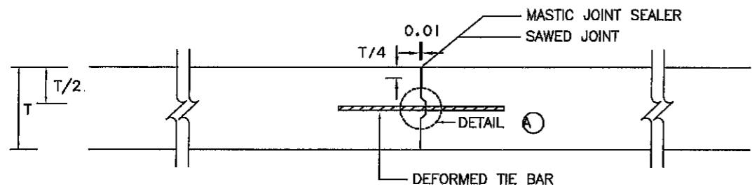
LONGITUDINAL JOINT
