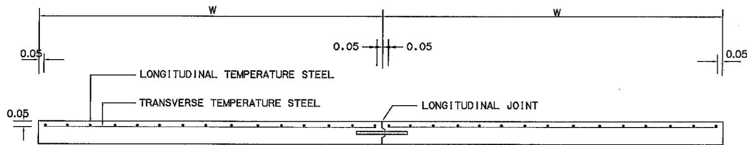
รูปตัดตามขวางพิจารณาจร คสล.
